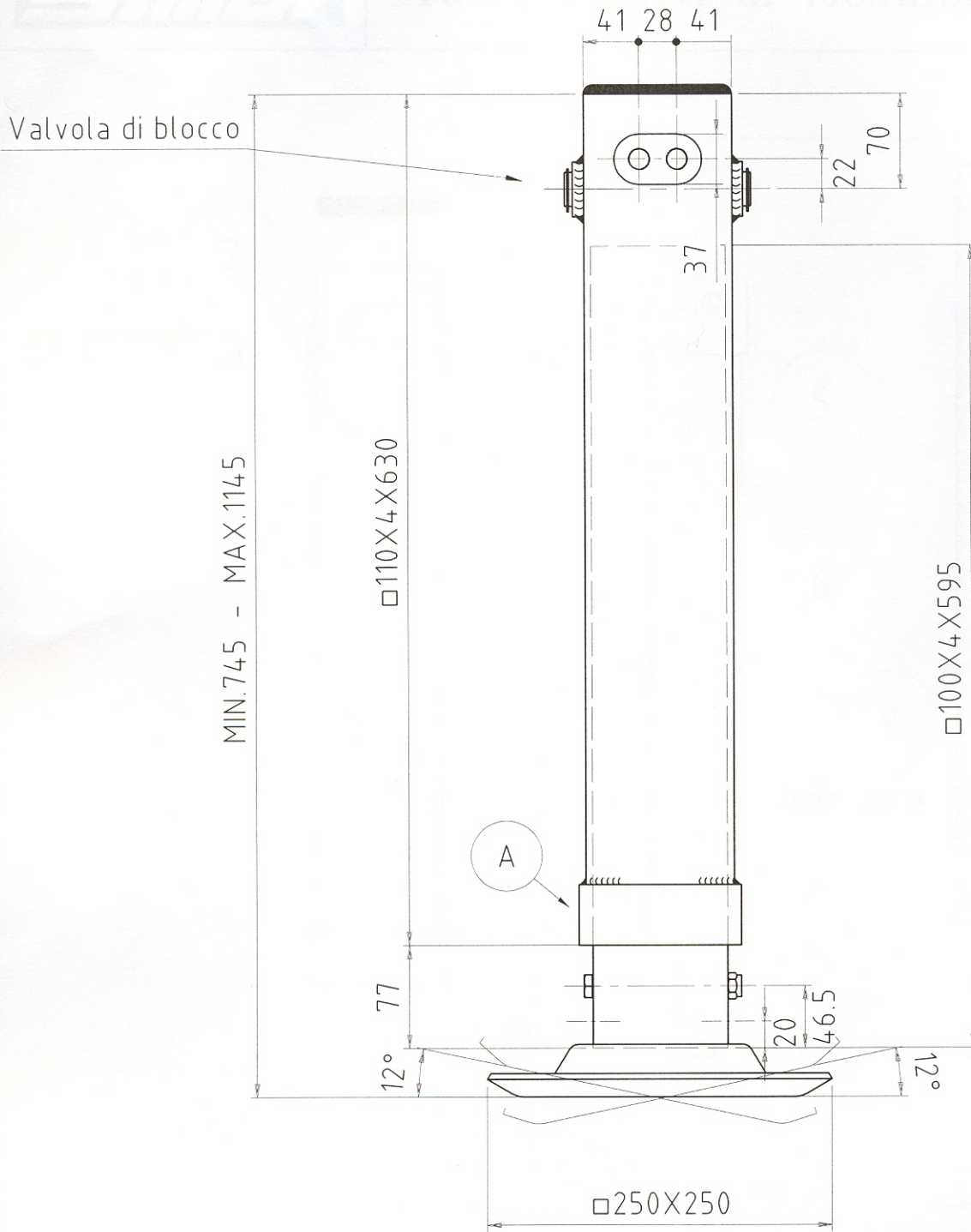
PIEDE D' APPOGGIO IDRAULICO CON VALVOLA DI BLOCCO
